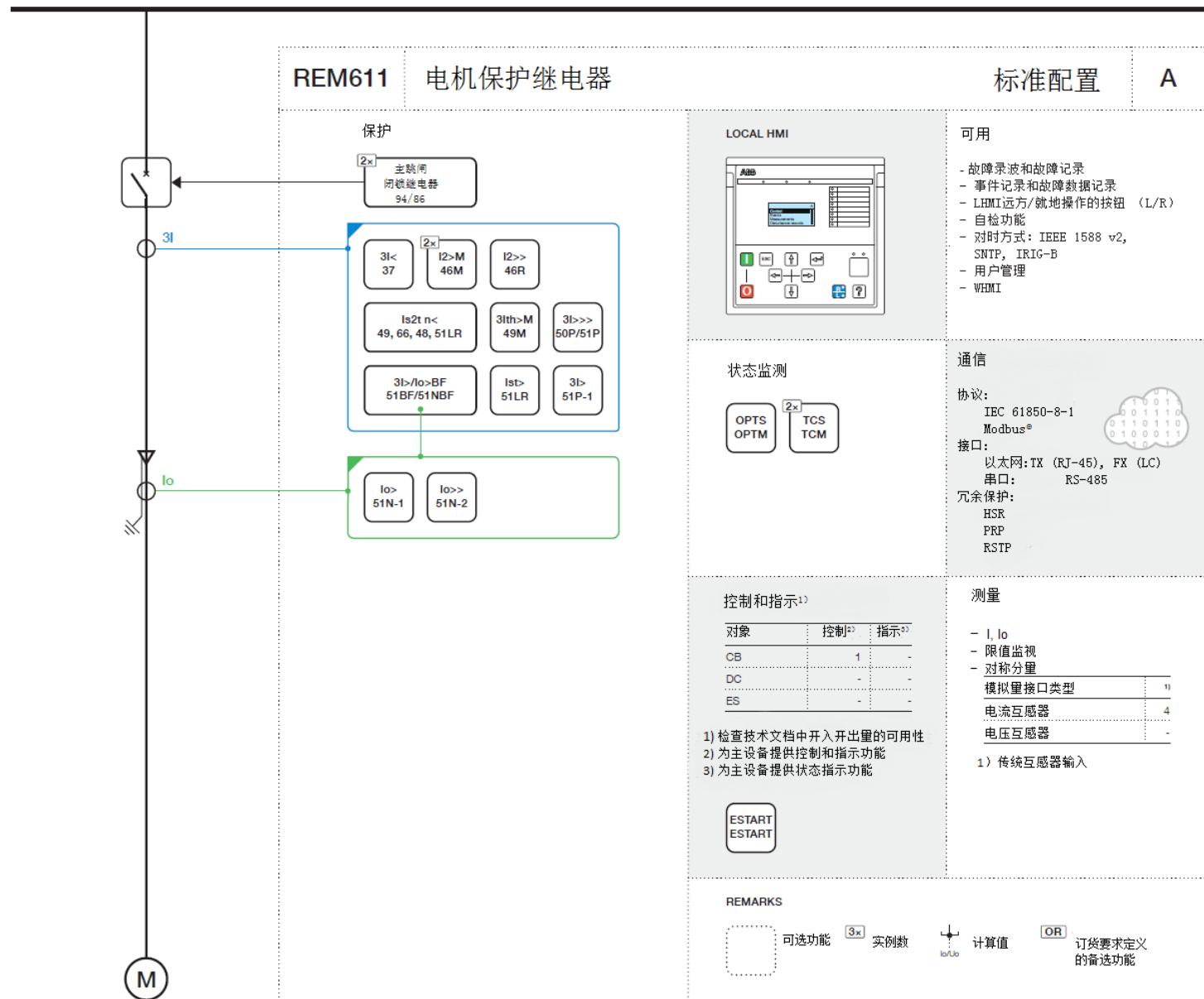
图1. 配置 A 保护功能总览
