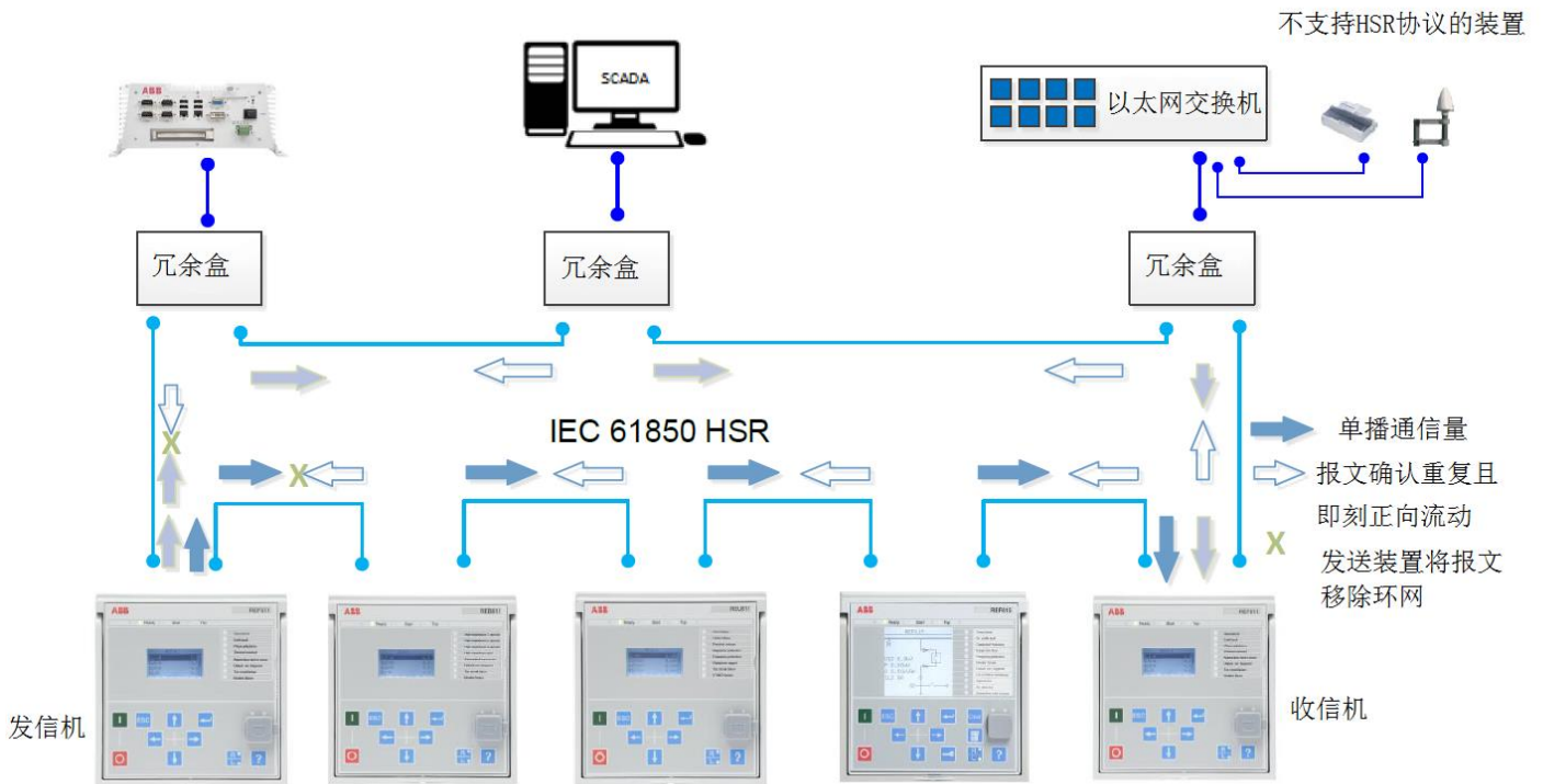
图5. 高可用性无缝冗余协议 (HSR) 解决方案
