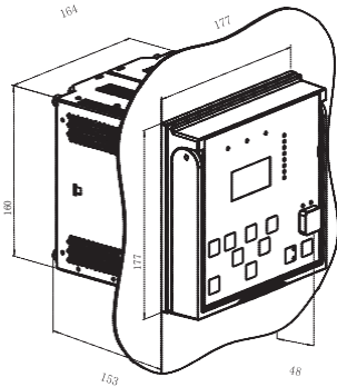
图8. 嵌入式安装
