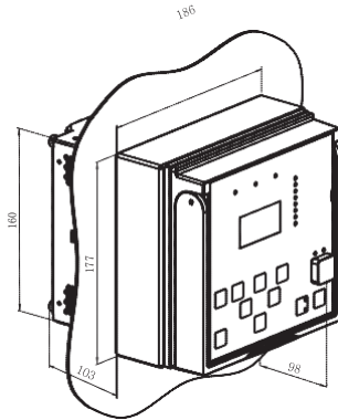
图9. 半嵌入式安装
