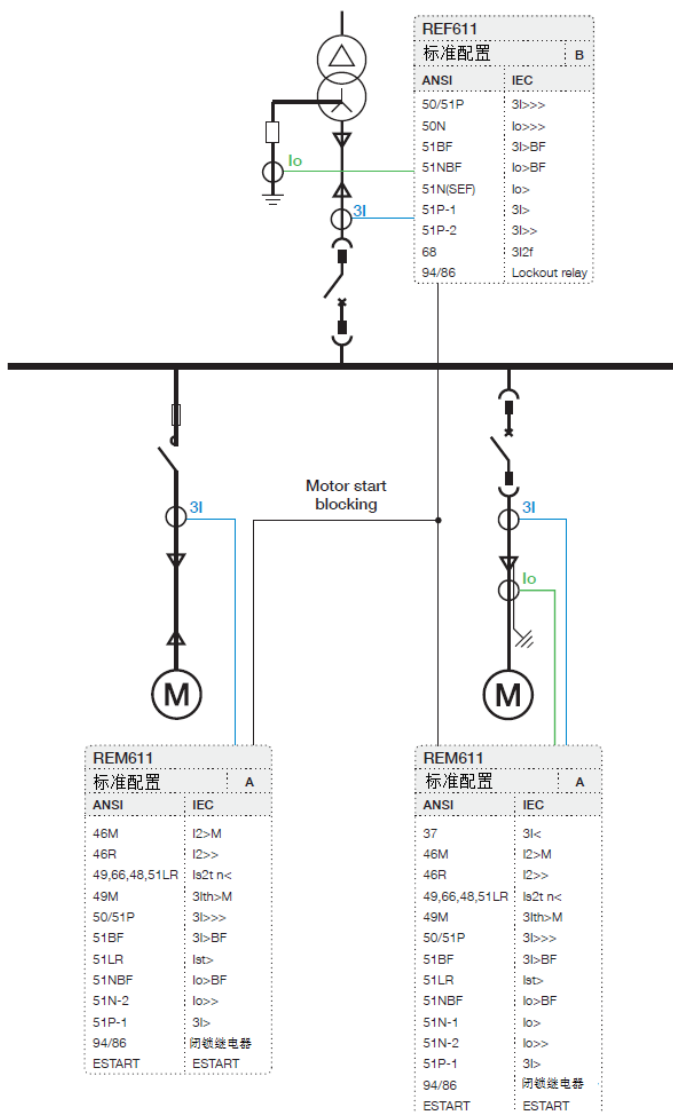
图2. 由接触器和断路器控制的电机基于标准配置A的保护和控制
